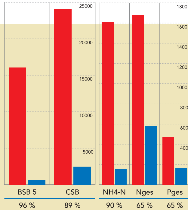
Wirkungsgrad 2002 Kläranlage Günsterode
