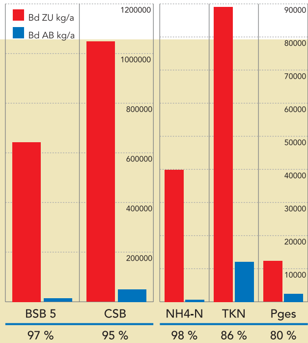
Wirkungsgrad 2002 Klärwerk Melsungen
